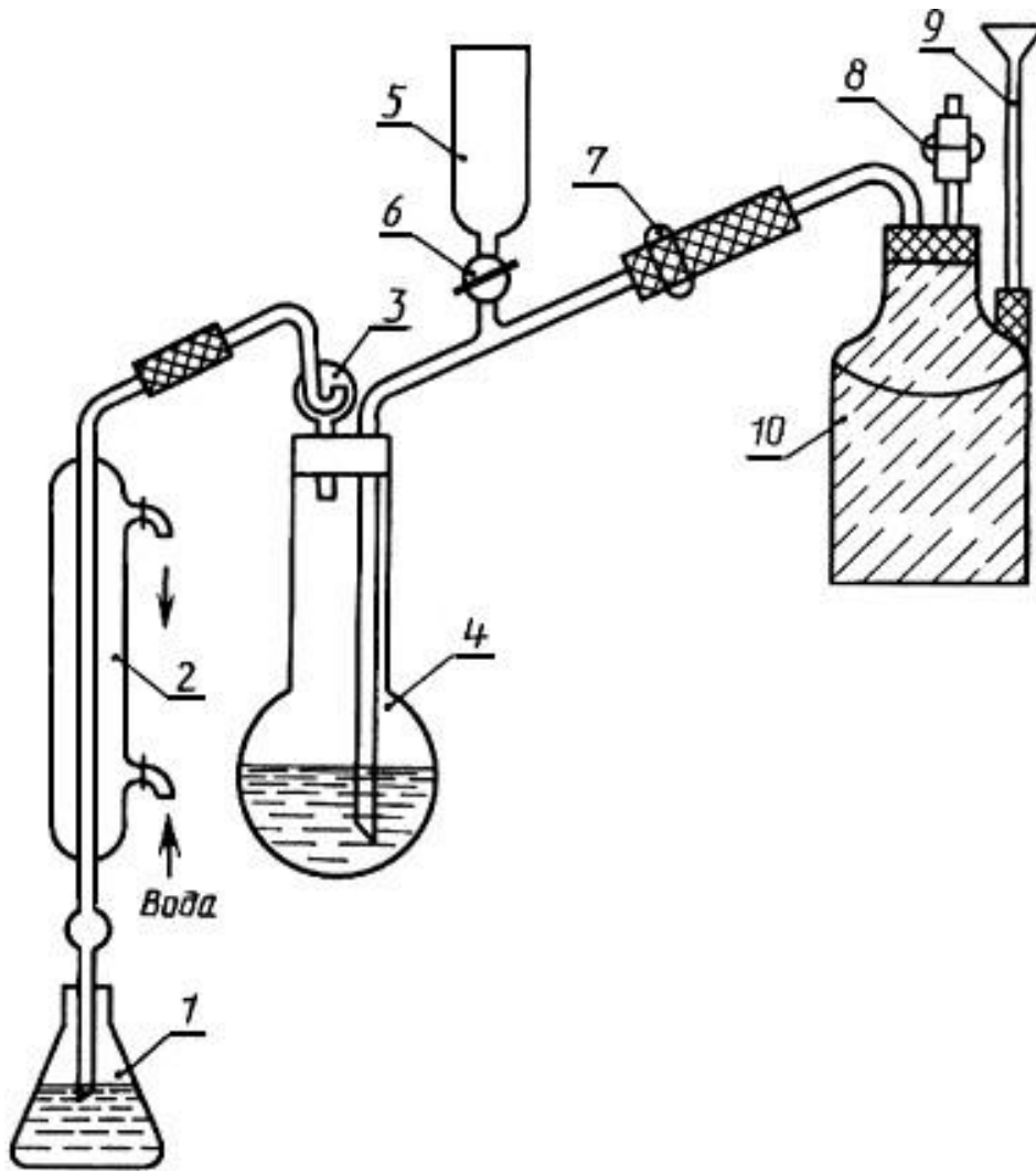
1 - приемная колба; 2 - холодильник; 3 - каплеуловитель; 4 - отгонная колба; 5, 9 - воронки; 6, 7, 8 - краны; 10 - паробразователь
